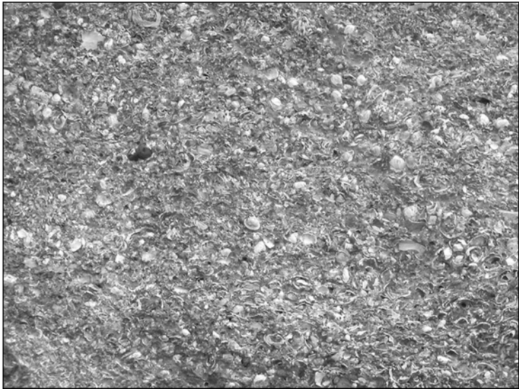
Corbula és Cirena kagylók sokasága a Fellegvári Homokkő Formációban
