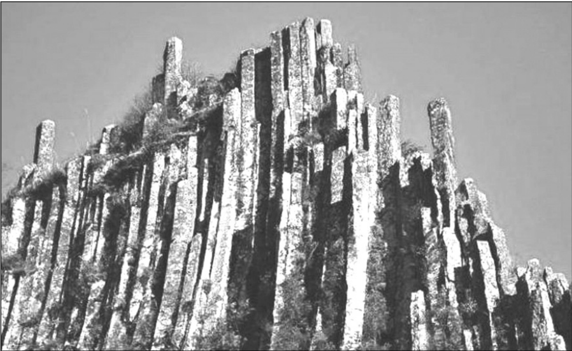
Páratlan látványt kínálnak a mohlepte bazaltoszlopok
